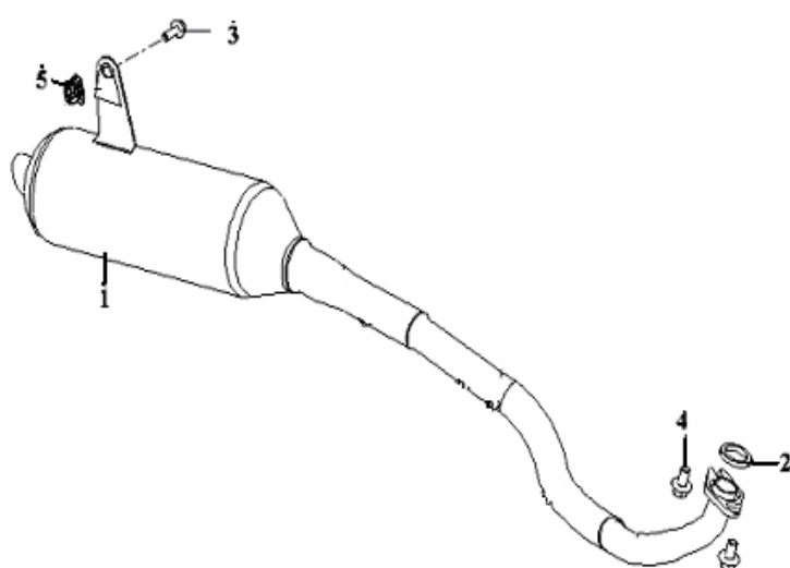
MUFFLER
